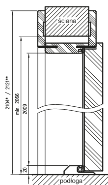
ościeżnica regulowana MDF
