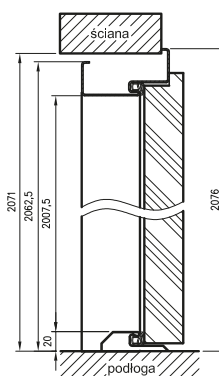
ościeżnica stalowa stała
