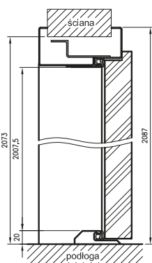
ościeżnica stalowa regulowana
