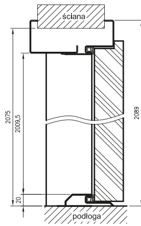
ościeżnica stalowa regulowana
