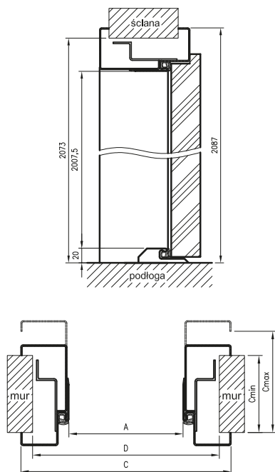
ościeżnica stalowa regulowana
